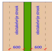
Samenstelling van een geleidelijn inclusief obstakelvrije stroken.
